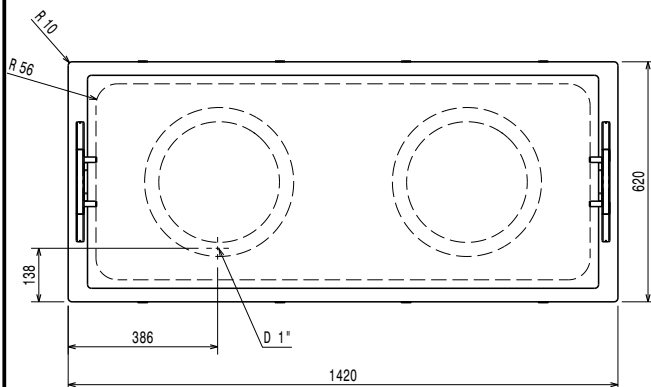
Boven aanzicht
